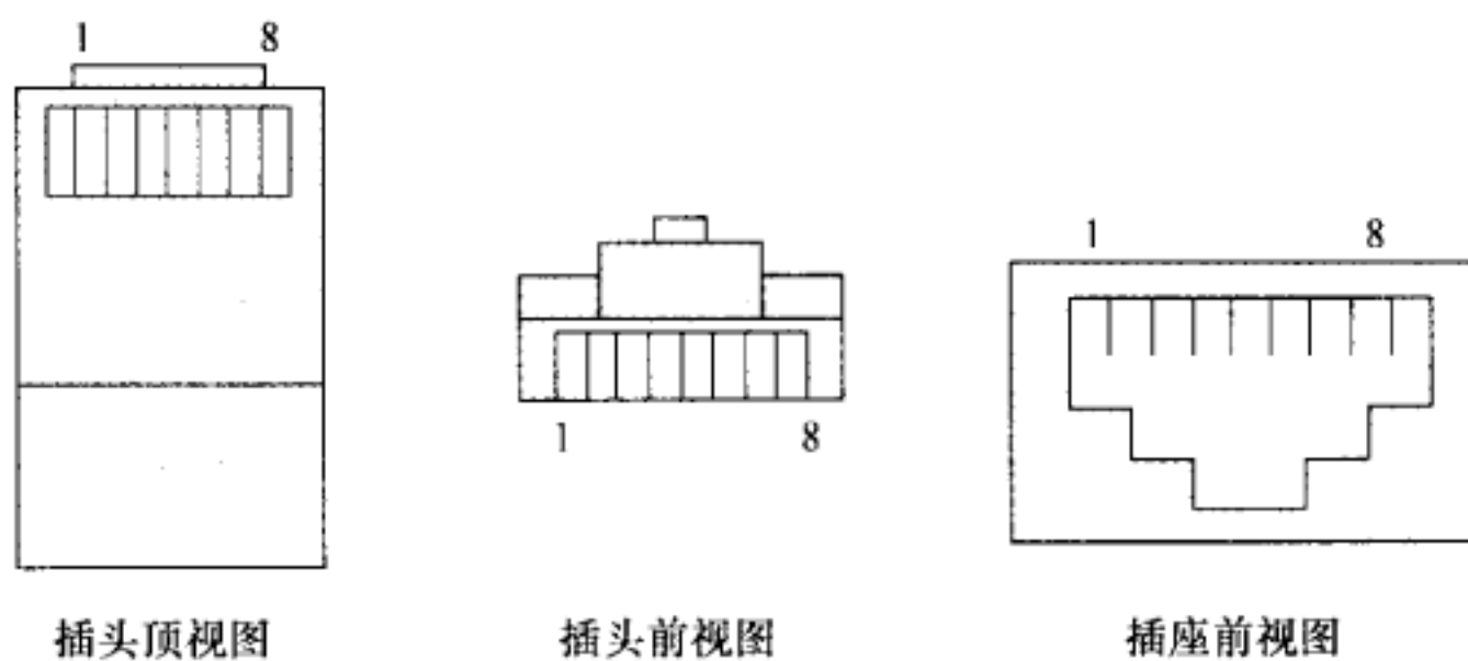
图 9.2.5 信息插座插头接线
