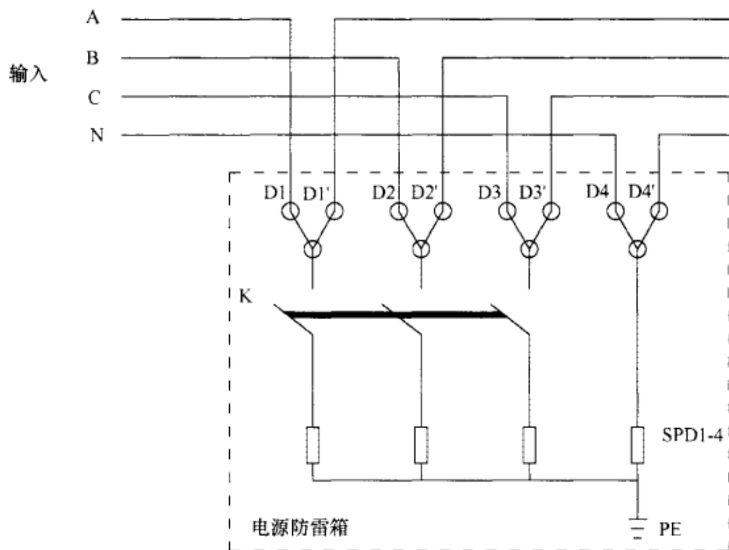
图1 V形接线
